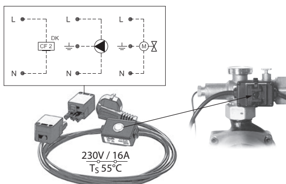
Электрическое подключение
