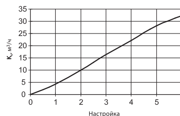
Расходная характеристика
