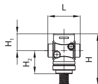
VGU DN 15-25
