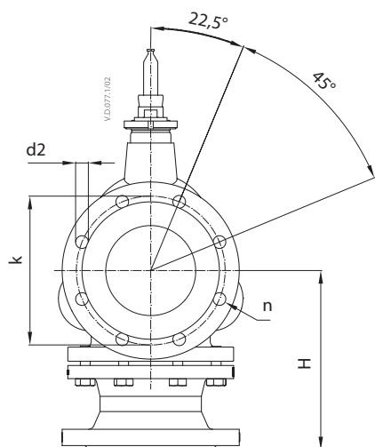
VF 3 DN 125-150
